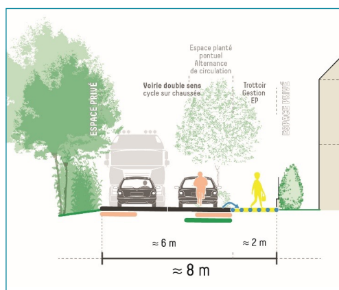
Coupe type de voirie : extrait du guide des espaces publics de Grenoble Alpes Métropole
